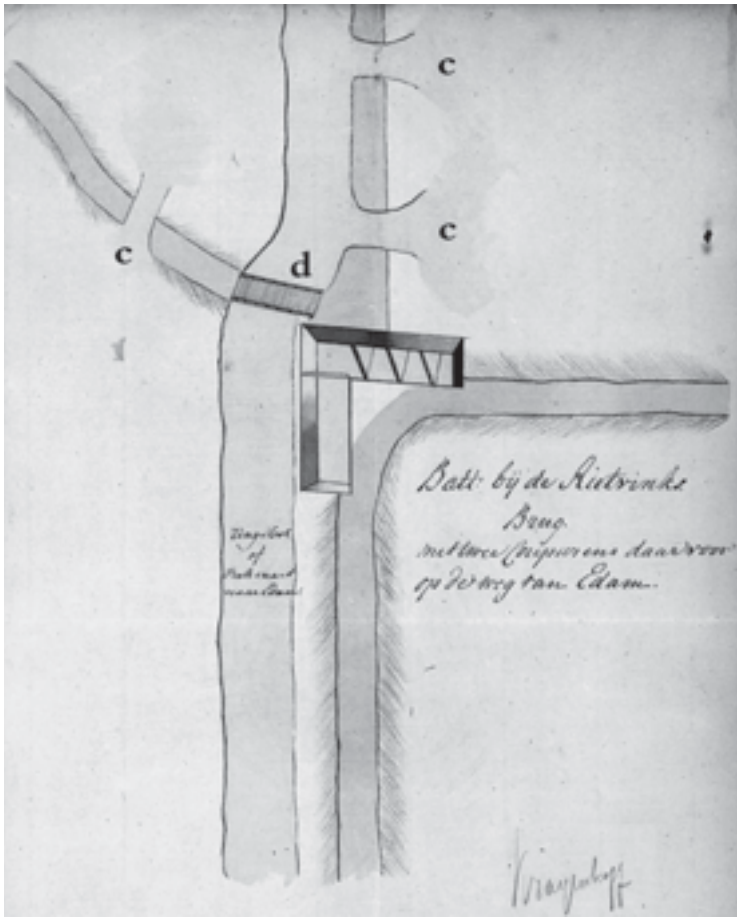
Afb. 4. Plattegrond van een batterij even benoorden Monnickendam. Door de coupures (c) in de kade loopt het water uit de ringsloot van de Purmer de Katwouderpolder in. Let ook op de doorgraving (d) in de naar de batterij lopende weg (Algemeen Rijksarchief, Familie-archief Krayenhoff, inv.nr. 6).
